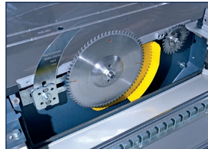
Detail mechaniky
