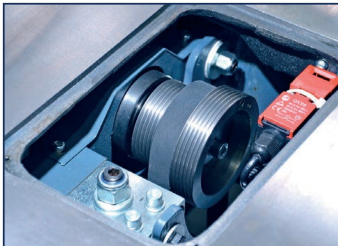
Změna otáček ve stole
