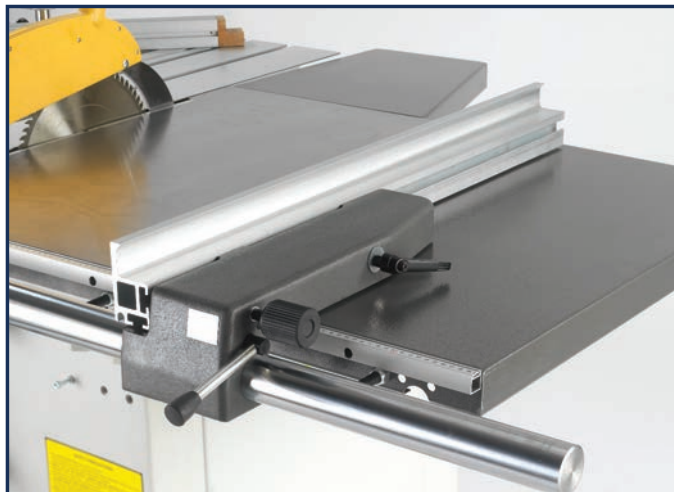
Litiné podélné pravítko
